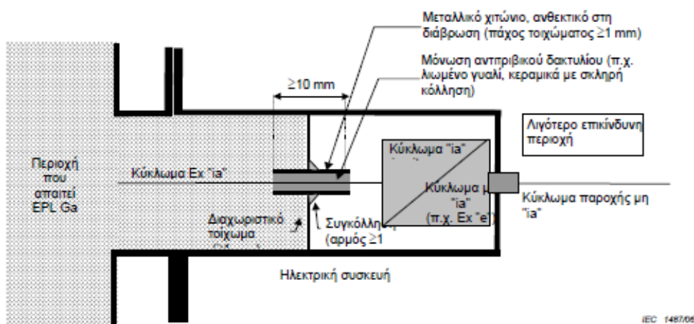
Σχήμα 1 – Παράδειγμα διαχωριστικού τοιχώματος με αντιτριβικό δακτύλιο αγωγών που θεωρείται ότι είναι αερόστεγές
